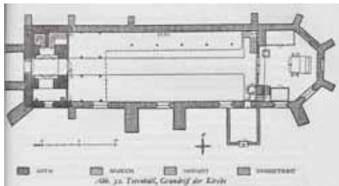
Kirche Grundriss
